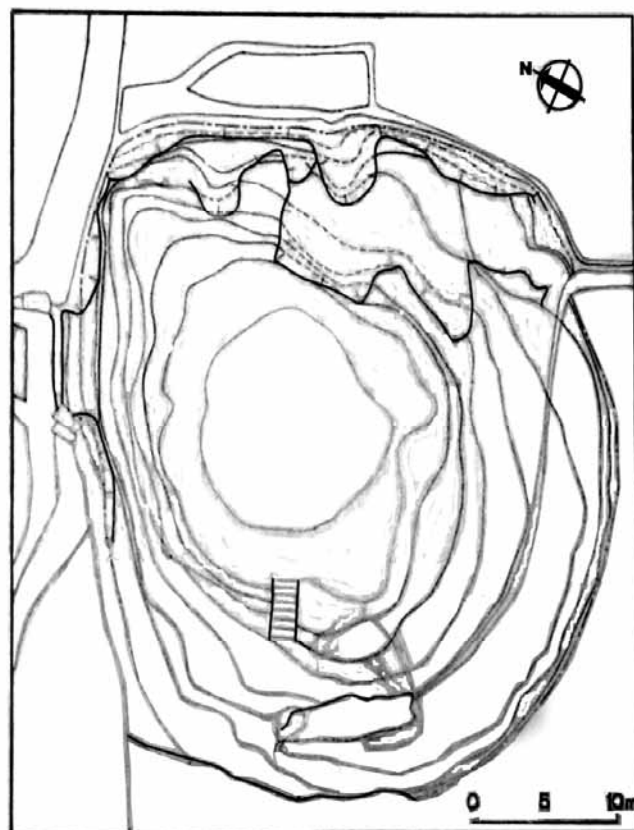
住蓮坊古墳実測図
