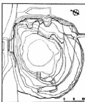
住蓮坊古墳実測図
